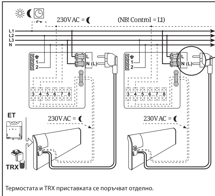
400V схема
